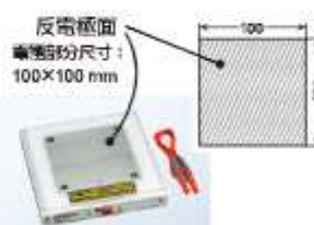
支持一體型反電極 (SM9001 附件)
