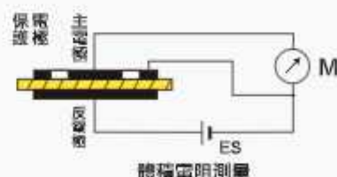
體積電阻測量
