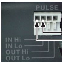
脈衝輸入端子
