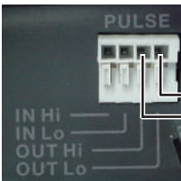
脈衝輸出端子
