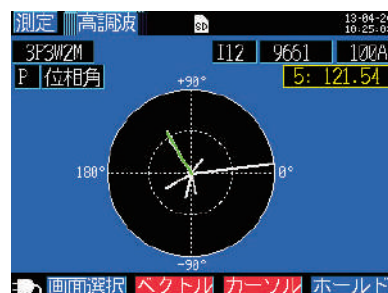
功率相位角向量畫面
